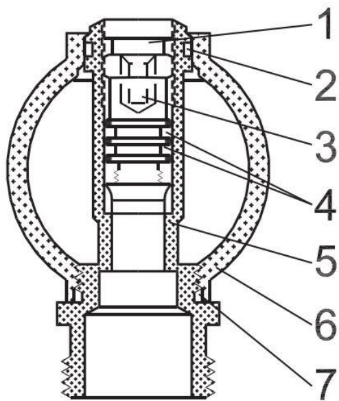
Рис. 1. Устройство подающей гребенки без расходомеров
