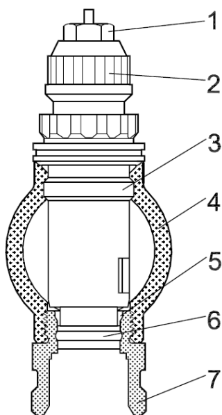
Рис. 2. Устройство обратной гребенки
