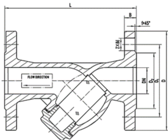
Габаритные размеры фильтров сетчатых типа ФСФ
