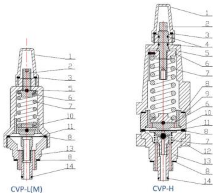
Рис. 1 – Конструкция
