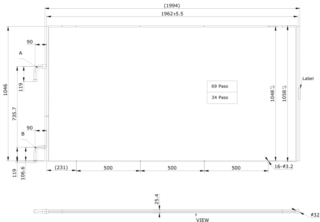
Габаритные размеры и изображение теплообменника микроканального модификации RC-2000.
