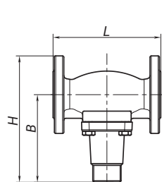
VFG-2R DN15–32
