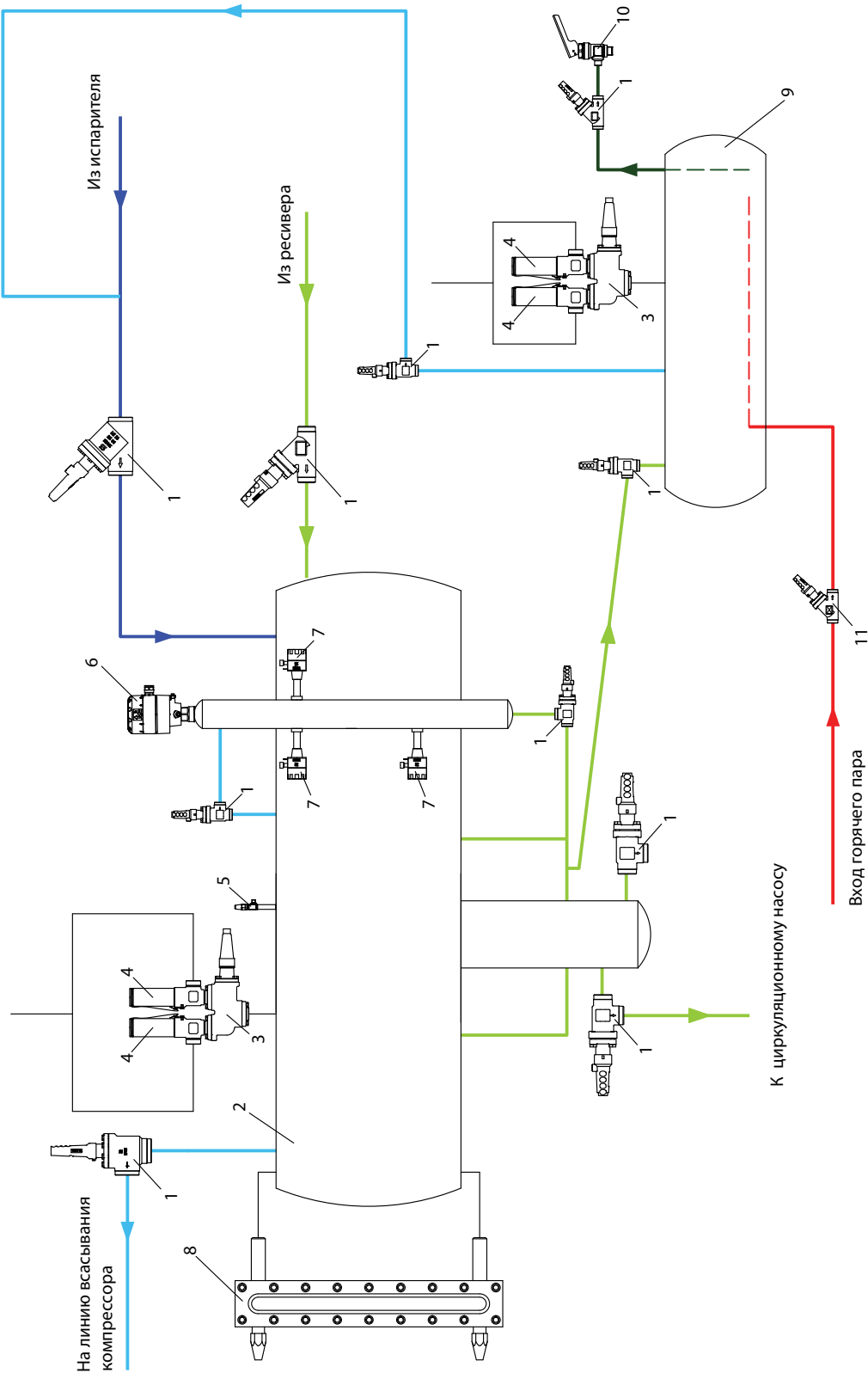
Схема №46. Слив масла из аммиачных систем охлаждения
