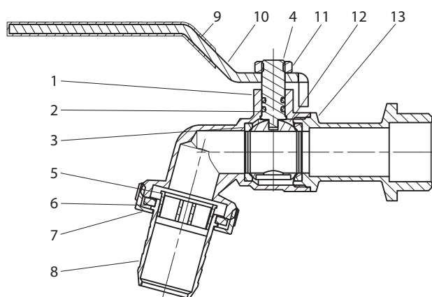
Кран шаровой латунный BVR-CR
