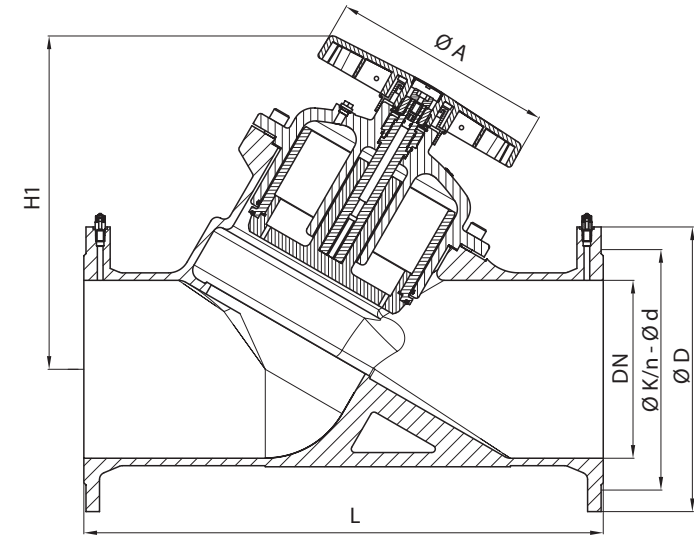
Клапан MNF-R2 DN200–400
