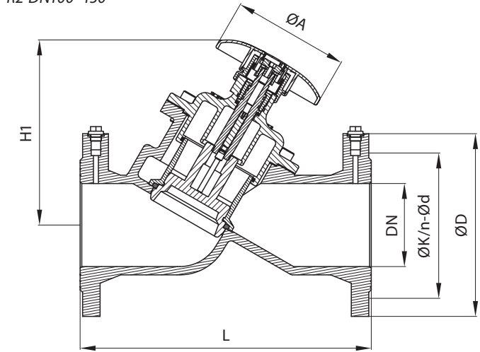
Клапан MNF-R2 DN100–150
