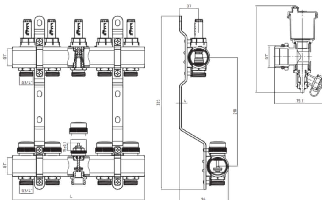
Рис. 1 - Коллекторы FHF-RF (коллектор для подающего трубопровода - сверху, коллектор для обратного трубопровода - снизу)
