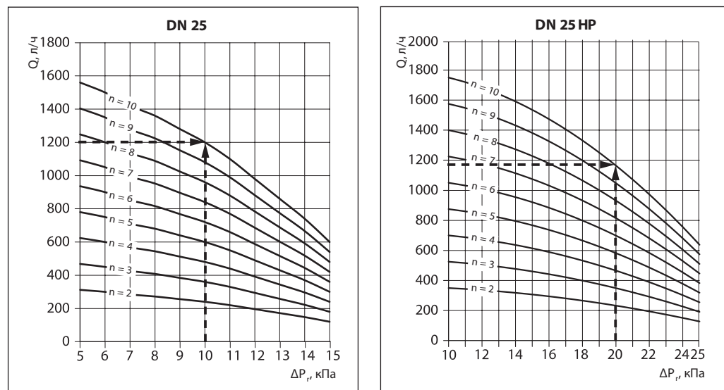
Настройки клапана APQT DN 25
