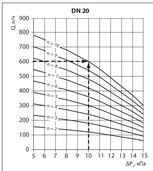
Настройки клапана APQT DN 20
