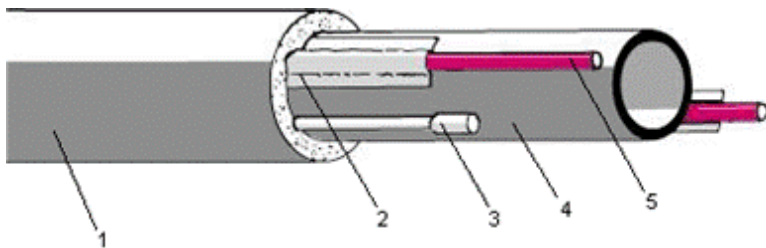
Рис. 4. Монтаж нагревательного кабеля ДЕВИ Flex-10T на металлической водопроводной трубе.
