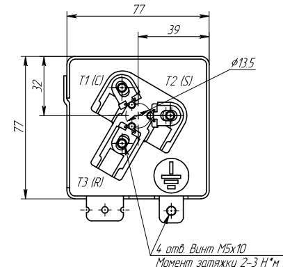
Клеммная коробка (1.1)
